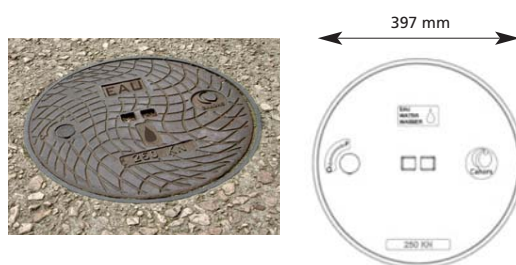
Poklop pro zatížení do 25 t
