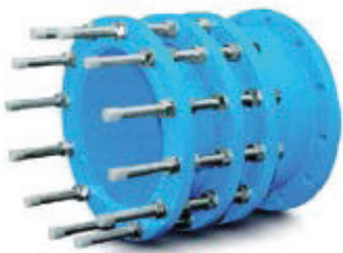
Objednací číslo: 13901 DN50-1600 PN16-100
