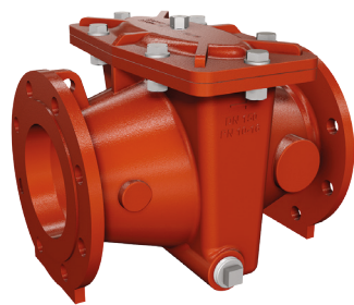
Objednací číslo: 10003 • DN40 - 1400 • PN10 - 40 Přírubový filtr s vrchním šišťením síta CLA-VAL Materiál: GGG-50 Síto: 2mm; jiné na poptávku
